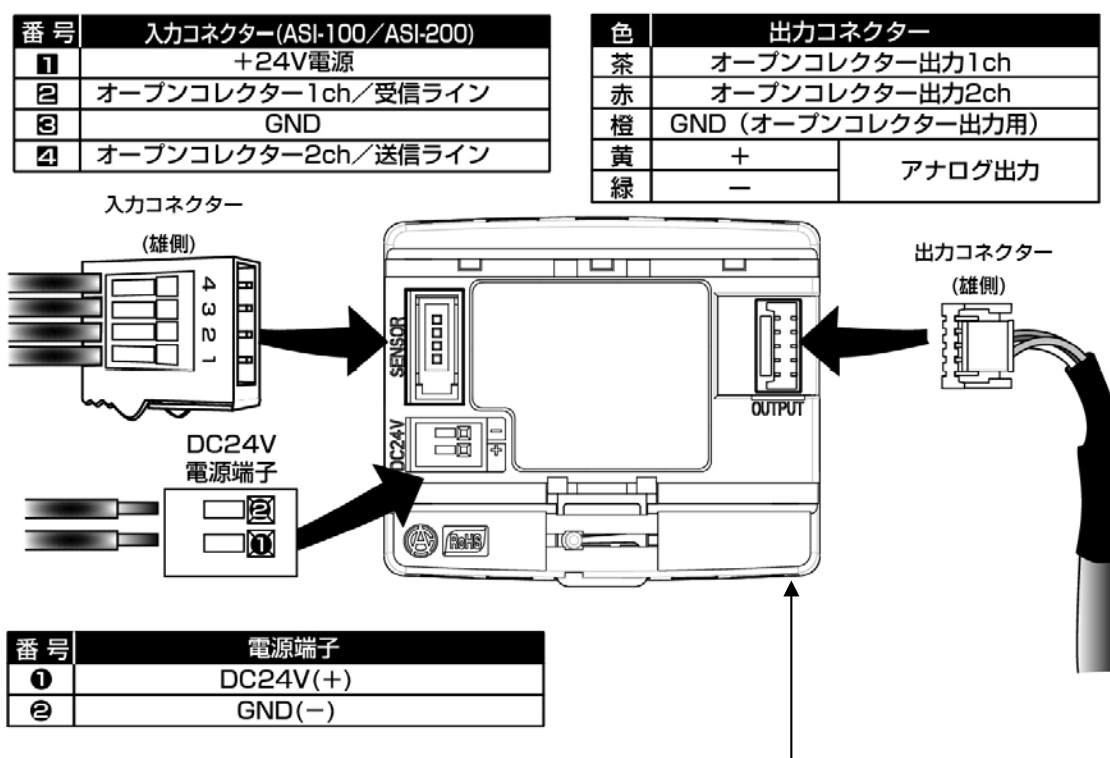
接続図
