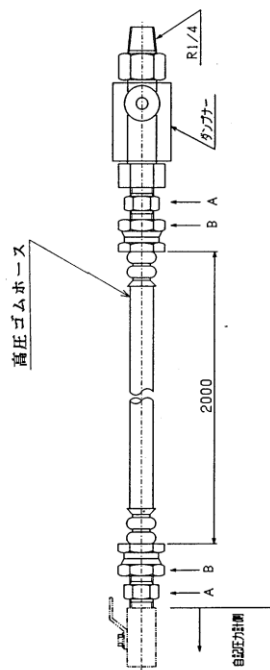
【図4】消火栓及び給水栓接続図
