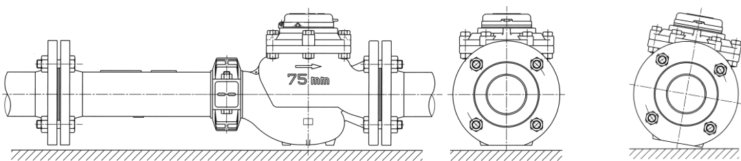
正しい据え付け方法
