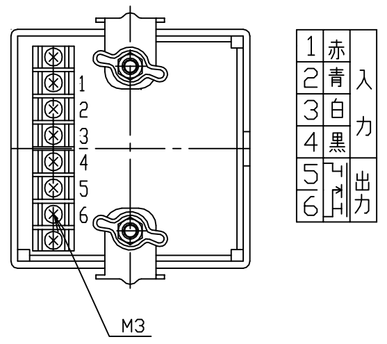
端子台説明
