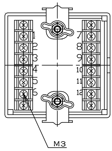
端子台説明
