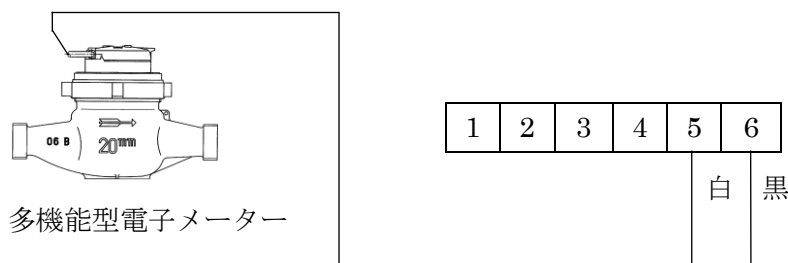
端子台結線説明図
