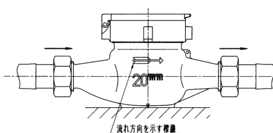
正しい据え付け方法
