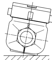
正しくない据え付け方法
