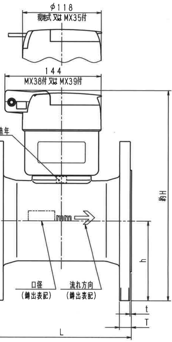
寸法表
