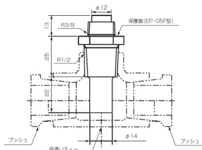
㊤保護管 (EP-05F 型)
