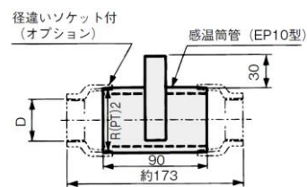
㊤感温筒管 (EP10, EP20～40 型)
