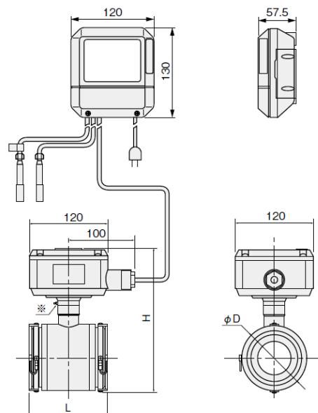
ウエハタイプ (ライニング：ふっ素樹脂)
