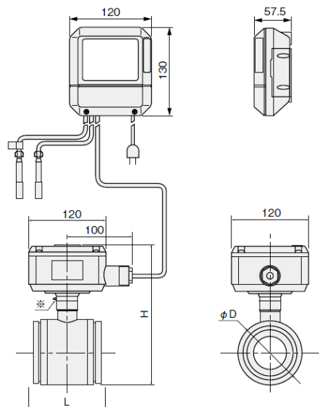
ウエハタイプ (ライニング：エポキシ樹脂)
