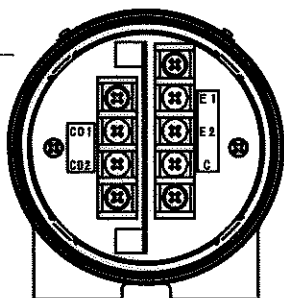
端子配置図
