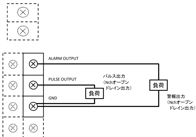
図 1 結線図【内蔵電池仕様】
