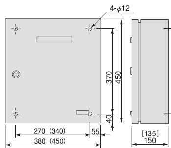
PR9A-4・PR9A-7・PR9A-2 *1 詳細は下表参照 単位:mm
