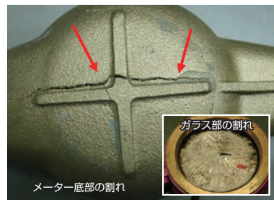
メーター底部の割れ
