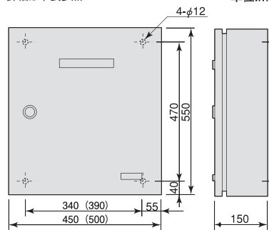
PR9A-7・PR9A-2 *2 詳細は下表参照 単位:mm
