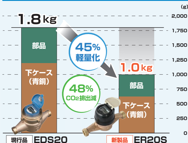
現行品 Eシリーズと新製品 ERシリーズの比較(当社比)
