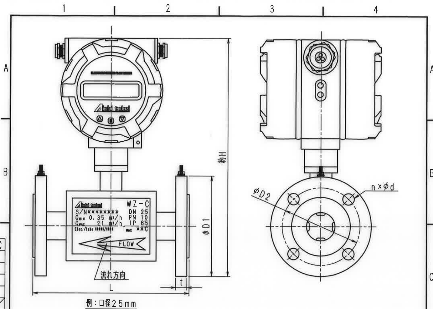
寸法表
